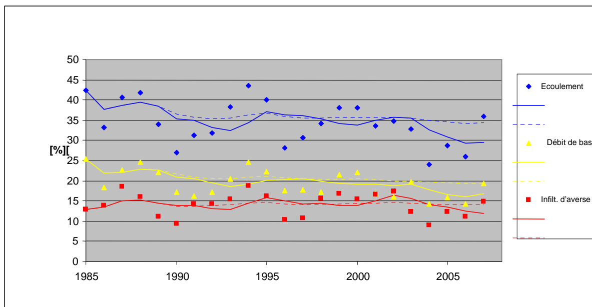
Illustration 40 : L'écoulement moyen exprimé comme pourcentage des précipitations zonales moyennes [%] de 5 sites de surveillance. Ligne complète : moyenne sur 5 ans ; pointillé : moyenne mobile.
