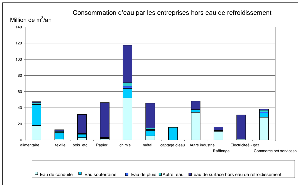
Figure 9 : Consommation d'eau par les entreprises (Flandre, 2003)
