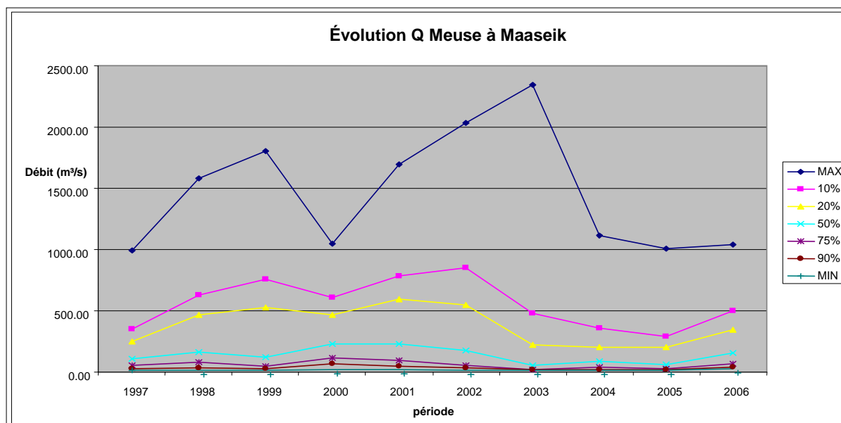
Figure 1: Meuse à Maaseik
