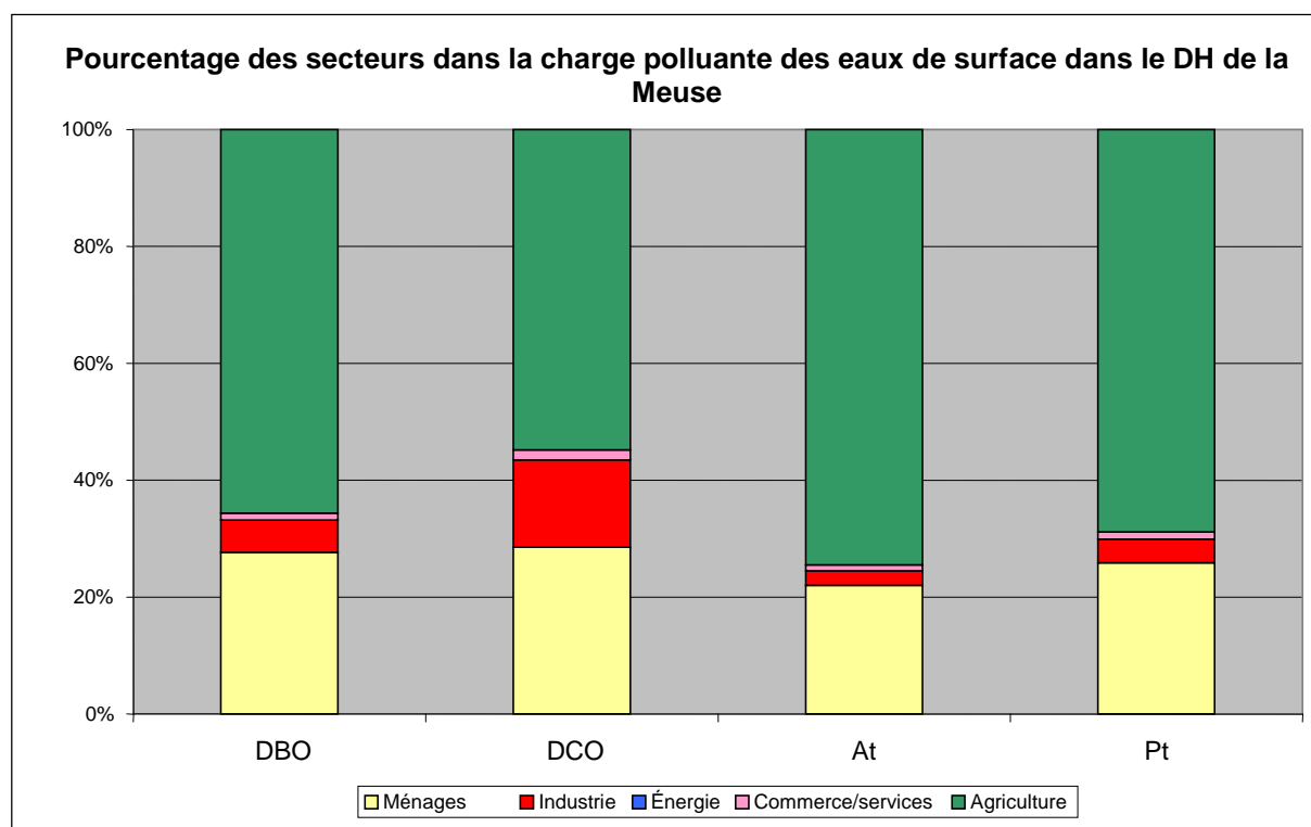
Figure 16 : Substances oxydables et nutriments : Charge nette (DH de la Meuse, 2005)
